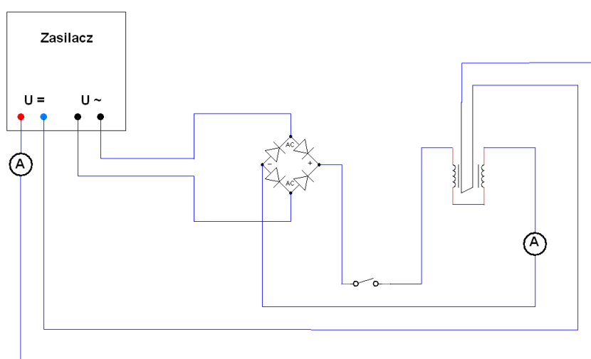
Rysunek E5.1. Schemat układu pomiarowego
